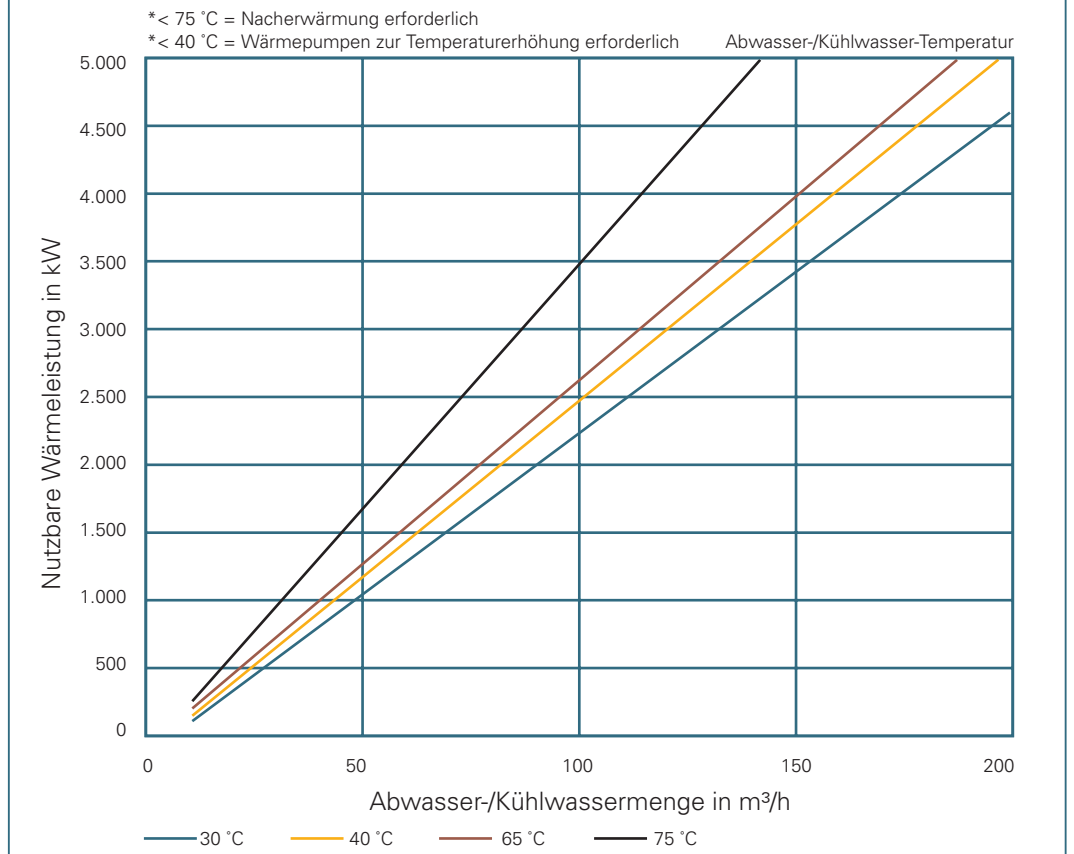
Bild 3.2_3: Anhaltswerte zur Abschätzung der nutzbaren Wärmeleistung von Kühl-/Abwasser-Abwärmenutzungsanlagen Abwasser-/Kühlwasser-Temperaturniveau 30 bis 75 °C
