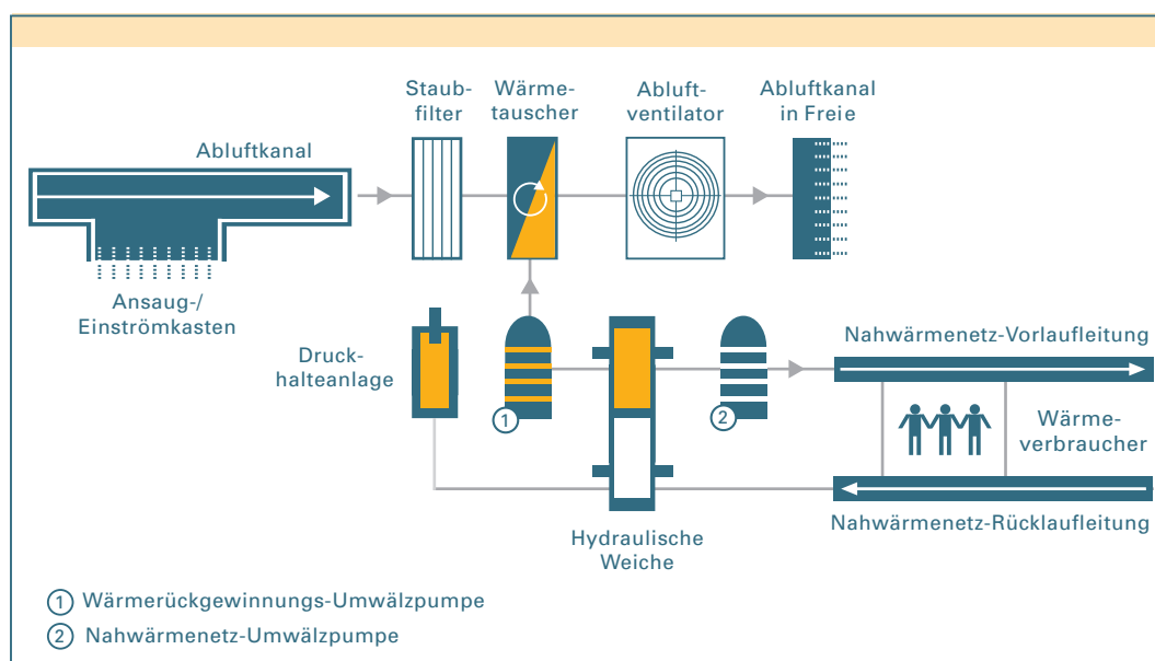
Bild 3.1_1: Übersichtsschema Abluftwärmenutzung
