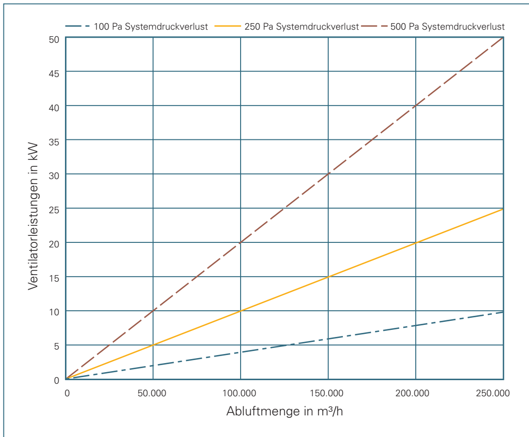
Bild 3.1_3: Anhaltswerte zur Abschätzung der Ventilatorleistung von Abluft-Abwärmenutzungs- anlagen
