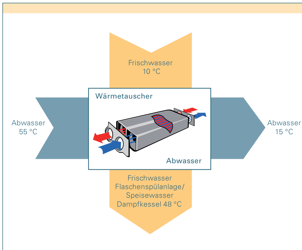
Bild 8.2_1: Übersichtsschema Abwasser- Wärmerückgewinnung (Quelle: www.s-i-z.de , leicht angepasst)
