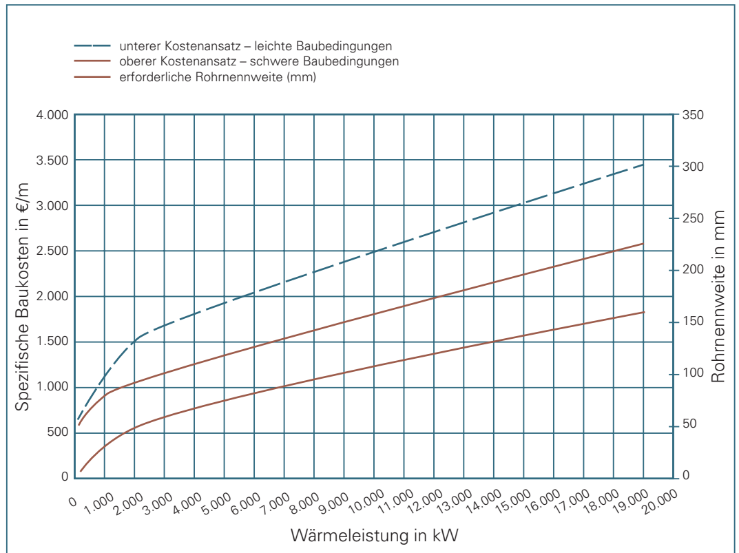
Bild 4.1_2: Kostenübersicht Nahwärmeleitungstrassen
