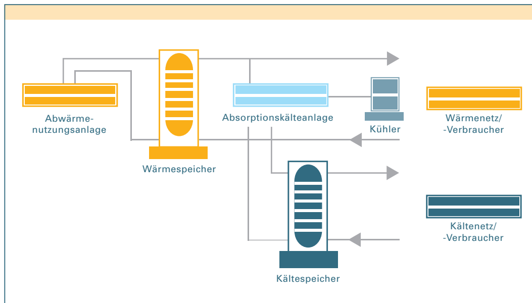
Bild 2.3_1: Übersichtsschema Abwärmenutzungssystem
