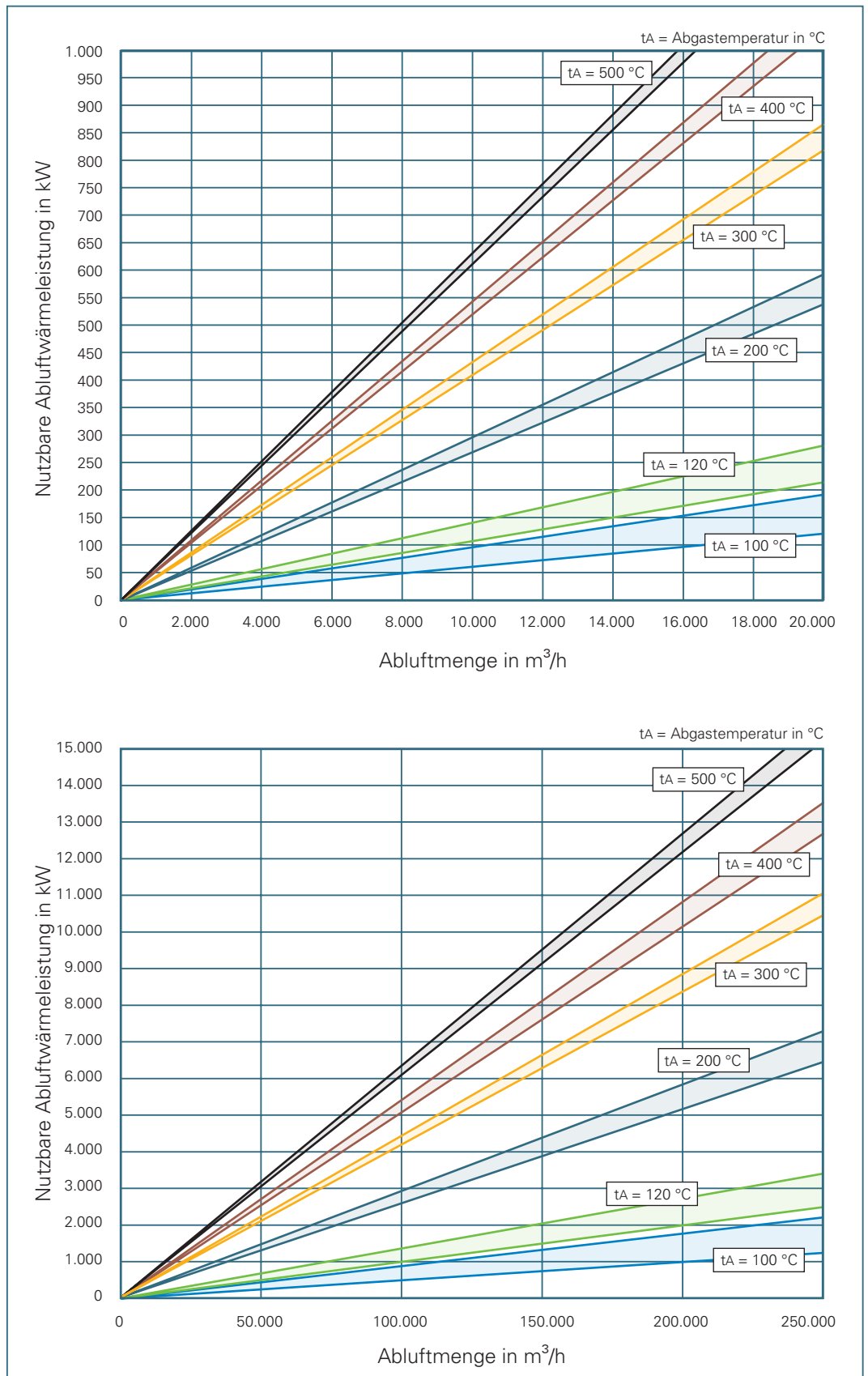
Bild 3.1_2b: Anhaltswerte zur Abschätzung der nutzbaren Wärmeleistung von Abluft-Abwärmenutzungsanlagen, Abluft-Temperaturniveau 100 bis 500 °C – Darstellung für größere Abluftmengen –
