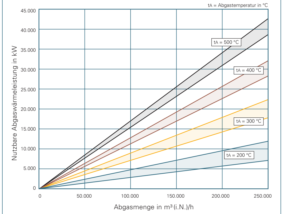
Bild 3.3_3b: Mögliche Wärmeleistungen bei Abgas-Abwärmennutzung als Anhaltswerte für Grob- analysen – oberer Lastbereich –
