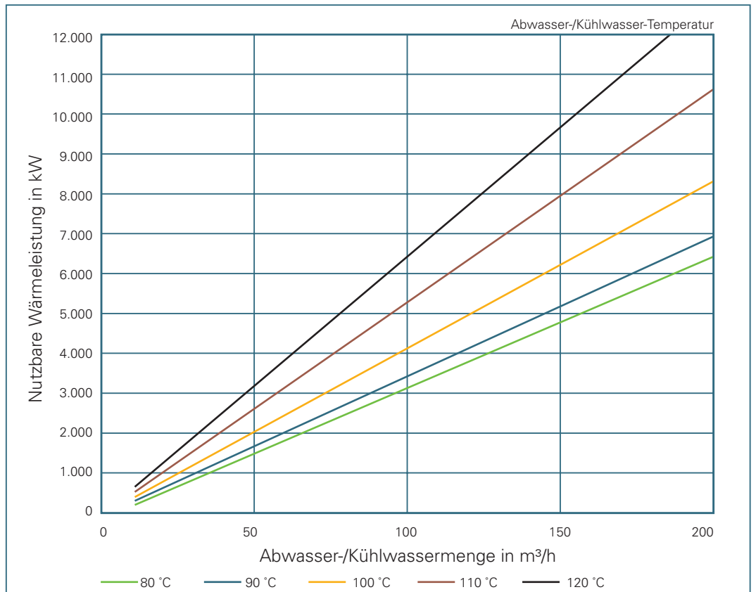
Bild 3.2_2: Anhaltswerte zur Abschätzung der nutzbaren Wärmeleistung von Kühl-/Abwasser-Abwärmenutzungsanlagen Abwasser-/Kühlwasser-Temperaturniveau 80 bis 120 °C
