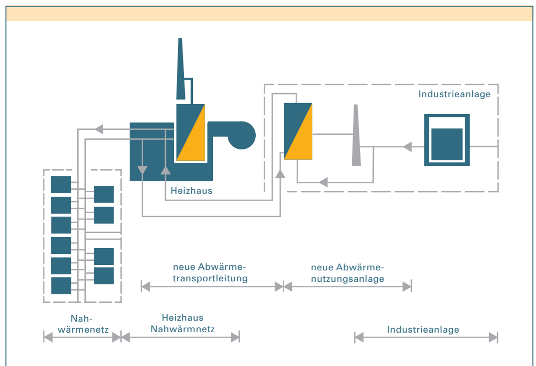
Bild 3.3_1: Übersichtsschema Abgas-Abwärmenutzung
