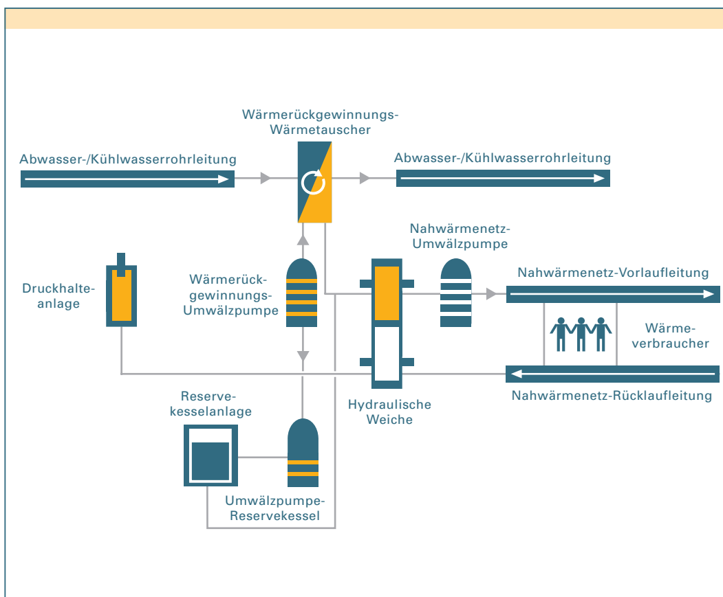
Bild 3.2_1: Übersichtsschema Kühl-/ Abwasser-Abwärmenutzung
