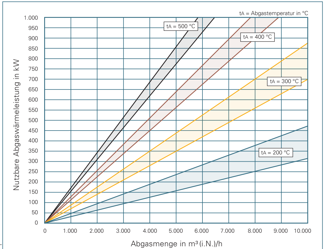
Bild 3.3_3a: Mögliche Wärmeleistungen bei Abgas-Abwärmennutzung als Anhaltswerte für Grob- analysen – unterer Lastbereich –
