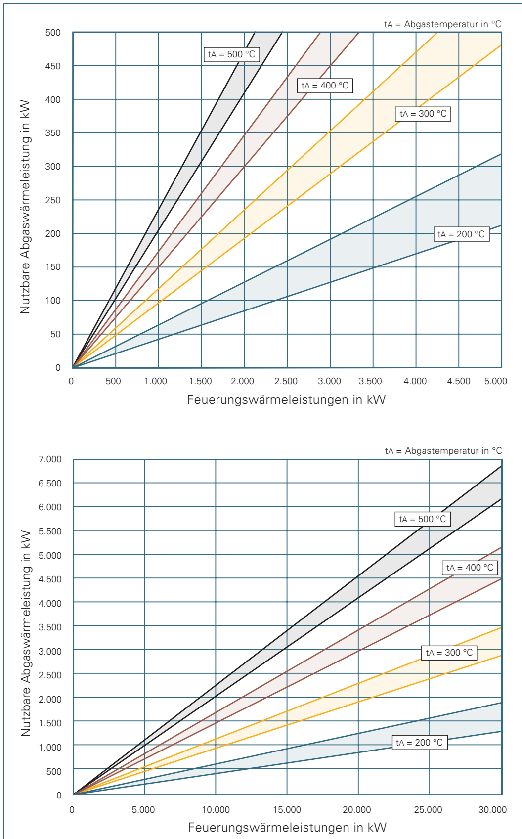
Bild 3.3_2a: Mögliche Wärmeleistungen bei Abgas-Abwärmennutzung als Anhaltswerte für Grob- analysen – unterer Lastbereich –
