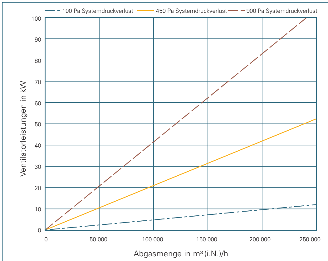
Bild 3.3_4: Ventilatorleistung von Abgas- Abwärmenutzungssystemen als Anhaltswerte für Grob- analysen
