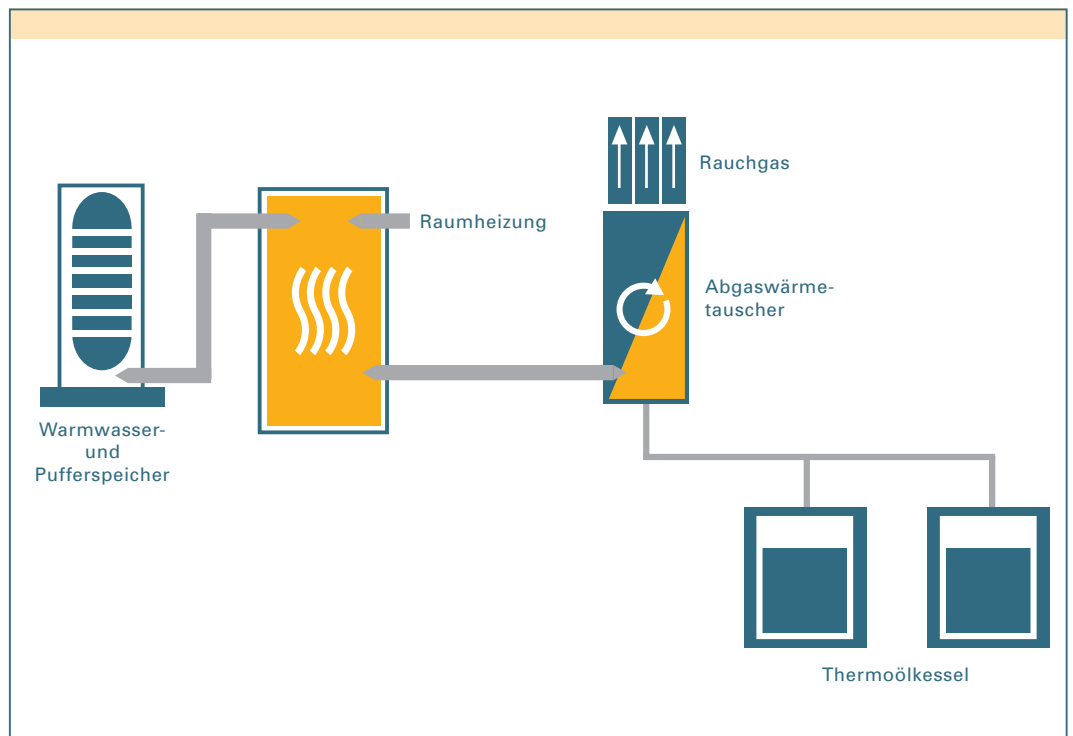
Bild 8.1_2: Einbindung der Wärmerückgewinnung (Quelle: TSB)
